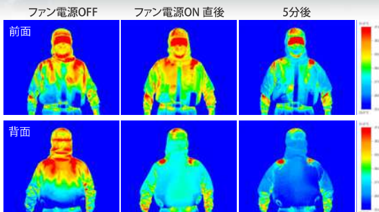
サーモグラフィー画像（ファン作動直後からクーリング効果あり）
